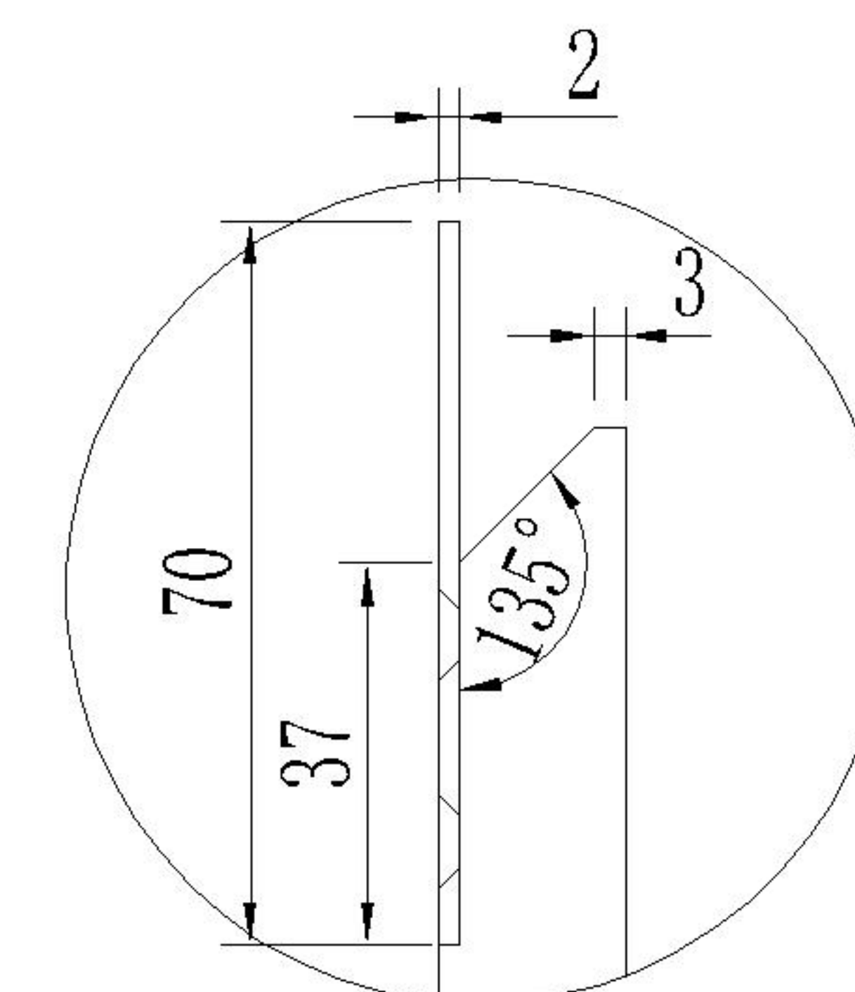
B处放大视图1:8
